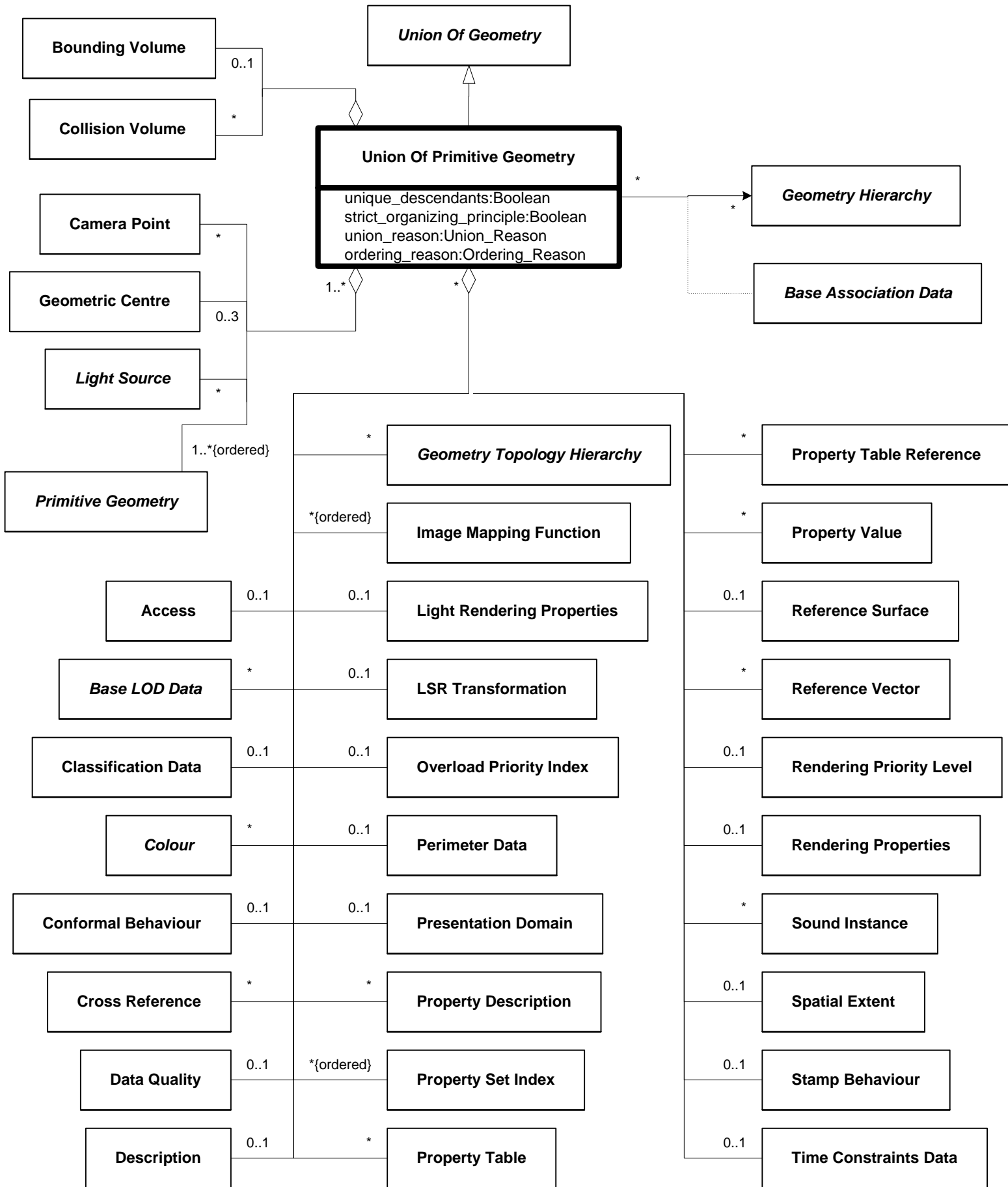
Figure 6.352 — DRM_Union_Of_Primitive_Geometry
